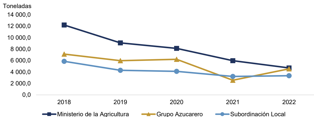
Gráfico 8.5- Consumo de combustible diesel por organismos seleccionados
